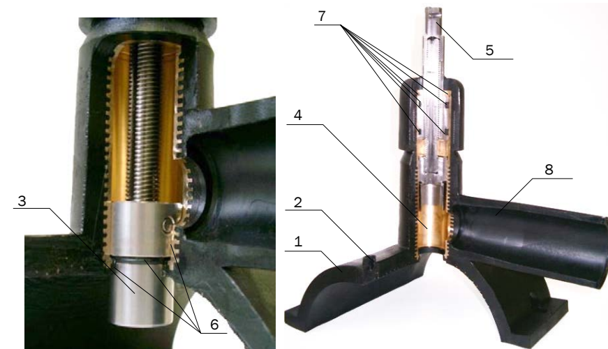
2 Конструкция вентиля для врезки под давлением Frialen, тип DAV: 1) корпус из полиэтилена PE100; 2) два контакта для сварки; 3) интегрированная фреза с верхним и нижним упорами; 4) металлическая гильза для хода фрезы; 5) вращающийся шпindel из легированной стали 1.4305 для управления приводом фрезы; 6) трехкратное внутреннее уплотнение в нижнем положении (ПЭ-металл, O-кольцо, металл-металл); 7) трехкратное внешнее уплотнение (O-кольцо); 8) выходной патрубков, рассчитанный на две сварки
